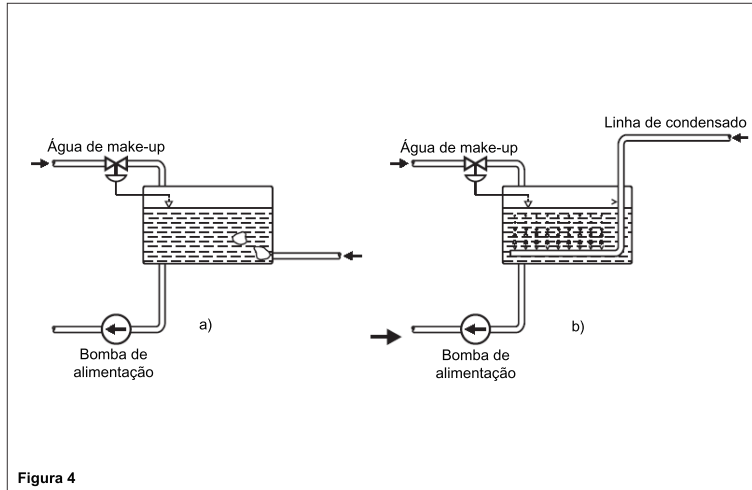
Fig. 4 - Como evitar o golpe de aríete quando alimentar condensado em tanques de água de alimentação.
