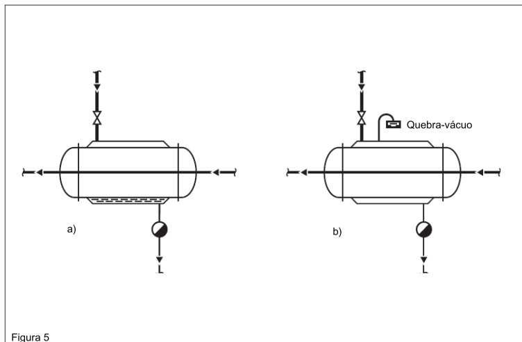
Fig. 5 - Como evitar o golpe de aríete em trocadores de calor onde o condensado se acumula pela formação de vácuo.
