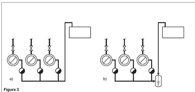
Fig. 3 - Como amortecer o golpe de aríete quando o condensado é elevado
