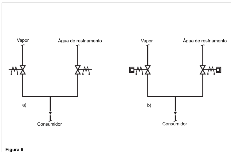
Fig. 6 - Como reduzir o golpe de aríete em plantas usadas em processos de aquecimento e resfriamento.
