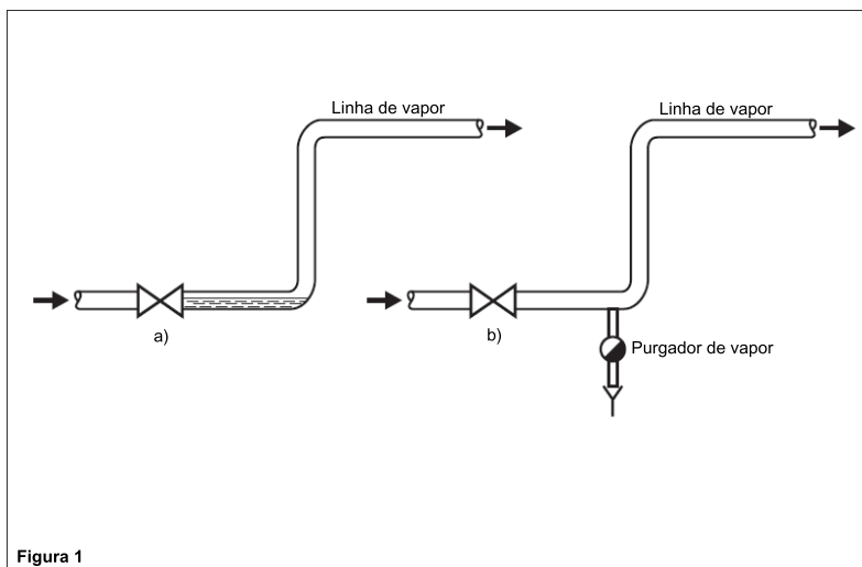
Fig. 1 - Como evitar golpe de aríete em linhas de vapor
