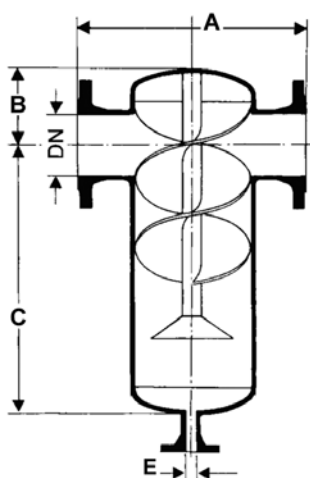
Separador Vertical
